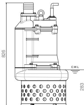
unit : mm Weight : 129kg
