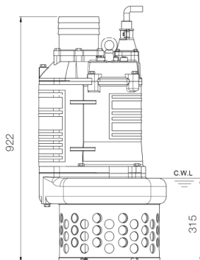
unit : mm Weight : 204kg
