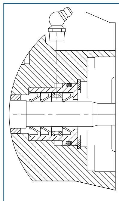
Fig. 304 – Lip seal
